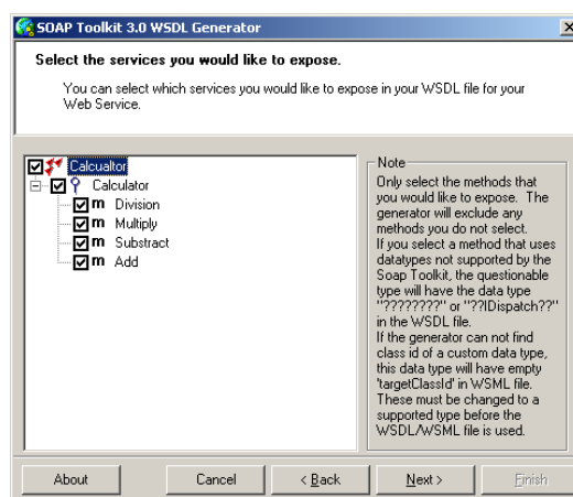
รูปที่ 1-6 หน้าต่างเลือก Method ที่ต้องการนำไป Deploy
